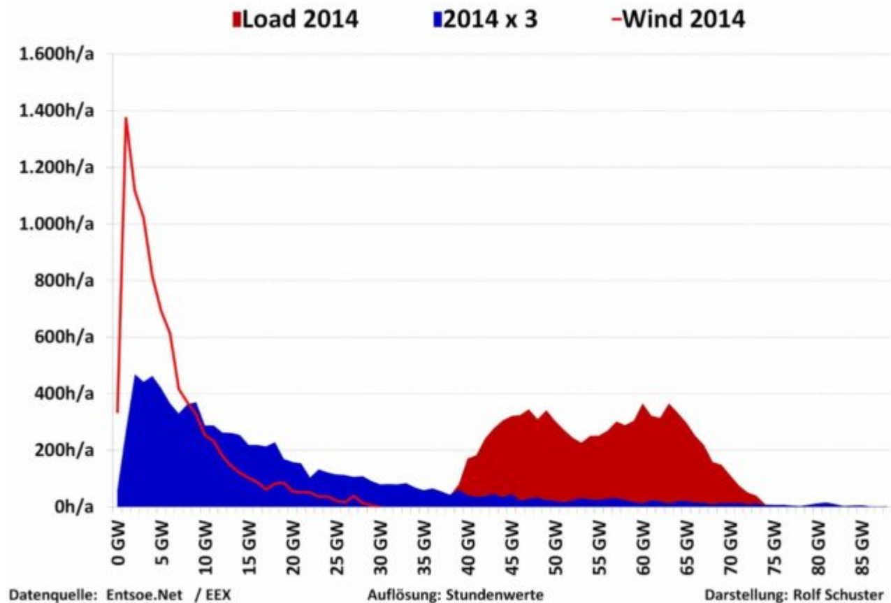
Abbildung 1: Häufigkeit von Windstrom- und Netzleistung
