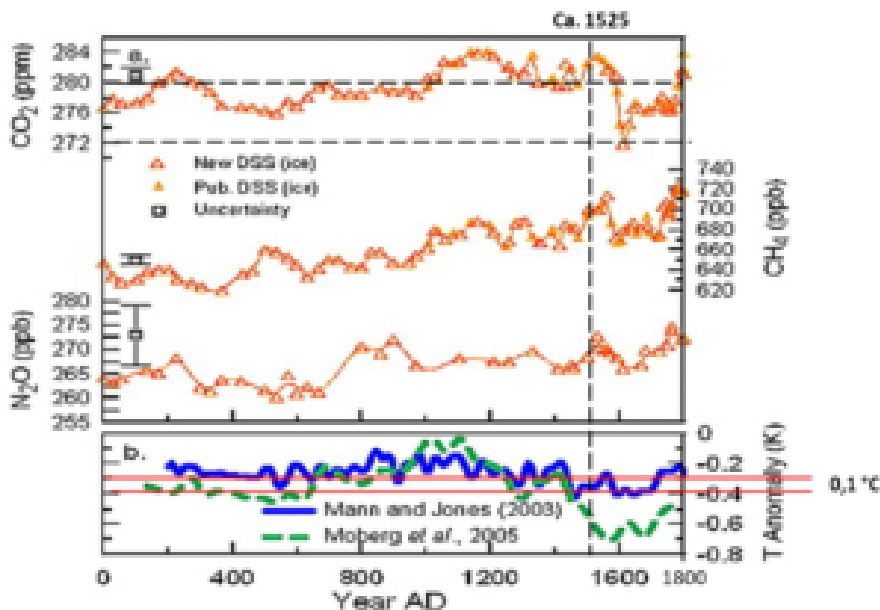
Bild 3 [7] Rekonstruktionen verschiedener Atmosphärogase vom Jahr 0 – ca. 1800
