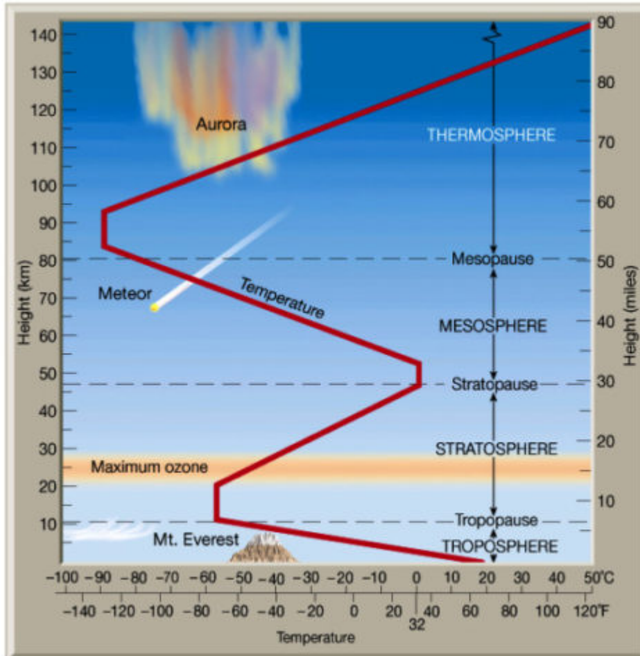
Abbildung 1: Vertikales Temperaturprofil der Erdatmosphäre. Man geht davon aus, dass mehr CO 2 die Stratosphäre abkühlt und die Troposphäre erwärmt. Der Betrag der Erwärmung an der Erdoberfläche wird wahrscheinlich um 1°C liegen bei einer Verdoppelung der CO 2 -Konzentration in der Atmosphäre. Quelle: Astrobites .
