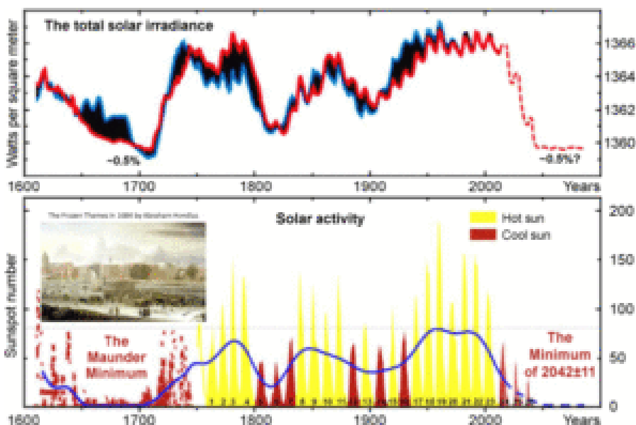
Abbildung 7: TSI-Variationen (mittels der rekonstruierten Daten [26]) und Sonnenaktivität seit 1611 [27] sowie Prognose von deren Variationen bis zum Ende des 21.
