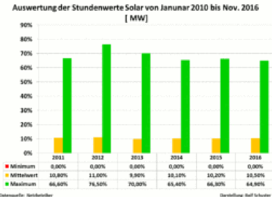
Bild 4: Kleinste, mittlere und größte Jahreseinspeisungen Sonne 2011 bis 2016
