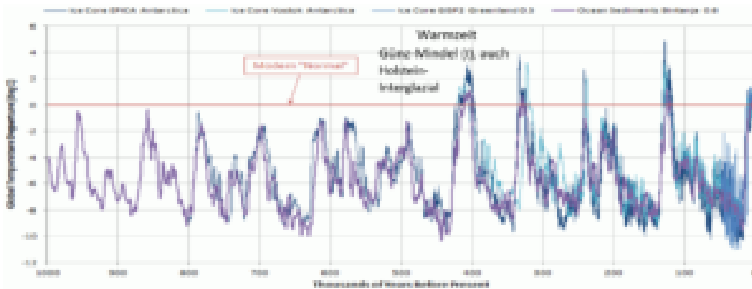
Bild 3 [3] Eiszeiten der letzten 1 Millionen Jahre. Die rote Linie kennzeichnet die aktuelle Temperatur Um einen ganz kleinen Eindruck der Zeit-Differenzen aufzuzeigen, hat der Autor aus Bild 2 und 3 Daten tabelliert:
