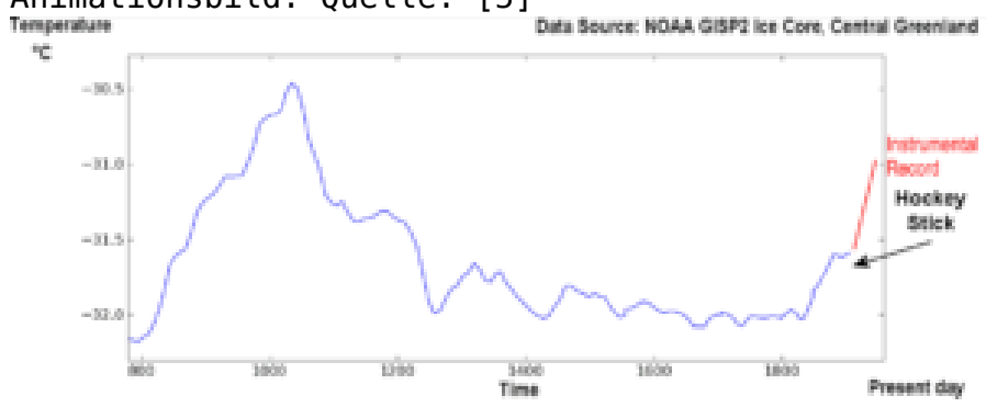
Bild 5.2 Globaltemperatur seit 800 n. Chr. Animationsbild. Quelle: [5]
