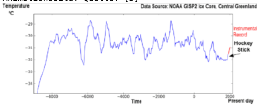
Bild 5.3 Globaltemperatur seit 8000 v. Chr. Animationsbild. Quelle: [5]
