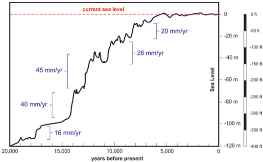
Bild 4 [7] Meerespiegel-Änderung der letzten 20.000 Jahre (Ende der Eiszeit)
