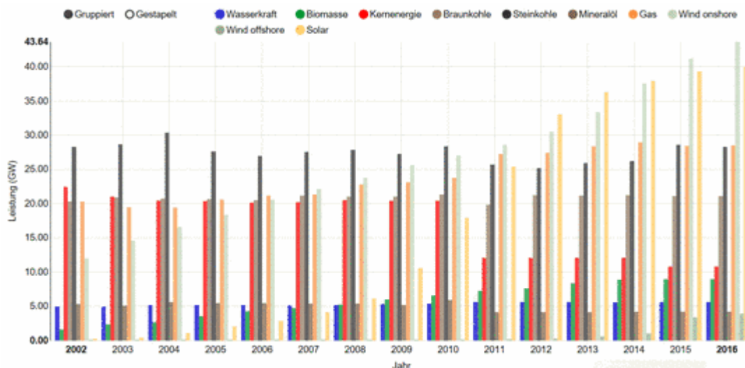
Bild 9 Installierte Nettoleistungen Deutschland gruppiert dargestellt.
