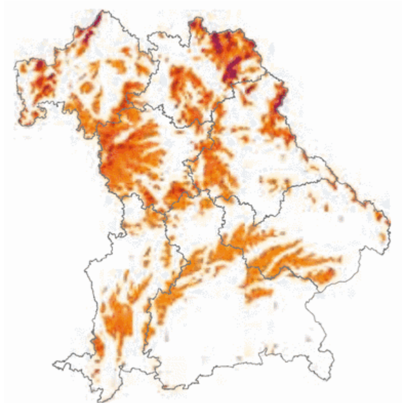
Bild 6 [3] Standorte in Bayern Anteil am Referenzertrag in 100 Meter Höhe. Die Farben zeigen den Anteil in Prozent. Quelle: Bayerischer Windatlas, Abb. 7
