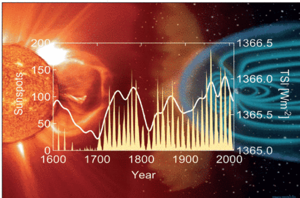
Abbildung 3: Sonnenaktivität während der vergangenen 400 Jahre. Weiße Kurve gibt die Total Solar Irradiance (TSI) an, die gelbe Kurve repräsentieren die
