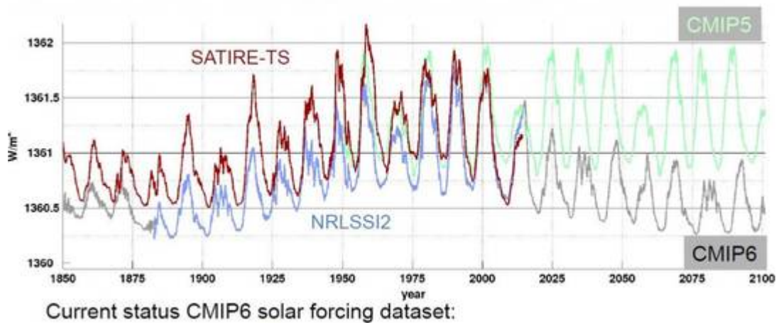
Abbildung 4: Neue und alte Kurven zur Sonnenaktivität während der vergangenen 165 Jahre. Quelle: Seite 9 in Matthes & Funke 2015 .
