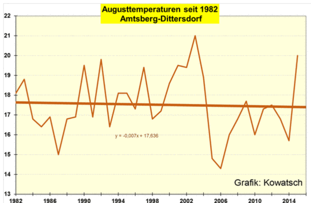
Abb.5: Das Ergebnis ist überraschend: Die Klimastation Amtsberg zeigt seit 1982 bis 2015 eine leicht fallende Trendlinie.
