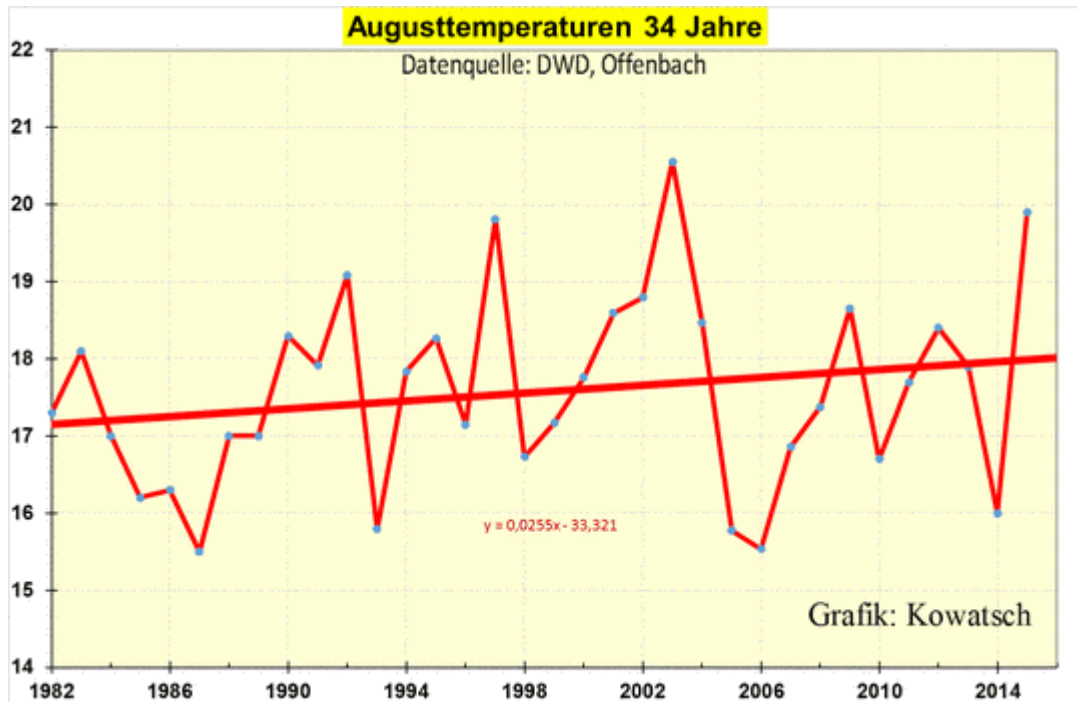
Abb.4: Die Augustmittel der deutschen Klima-Stationen des Deutschen Wetterdienstes (DWD) zeigen seit 1982 einen aufsteigenden Trend. Man könnte sagen, der August wurde in diesem Zeitraum um 0,8 Grad wärmer. Wie es weitergeht, weiß niemand. Stimmt diese Grafik wirklich?
