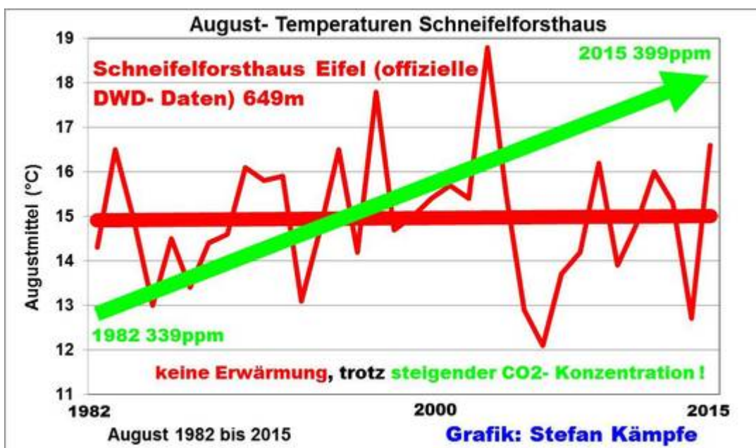
Abb. 3: Keine August- Erwärmung in der Eifel – trotz steigender CO 2 - Werte.
