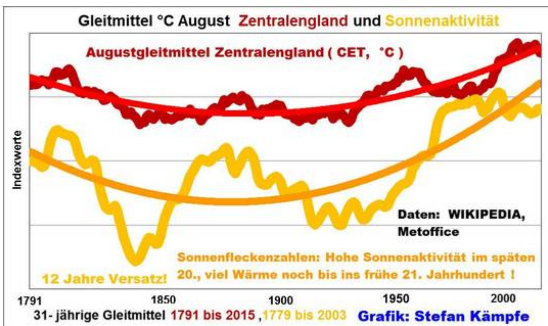
Abb.11: Mit gewissen Abstrichen besteht eine gute Übereinstimmung zwischen Sonnenaktivität (gelb, unten) und den Augusttemperaturen in Zentralengland
