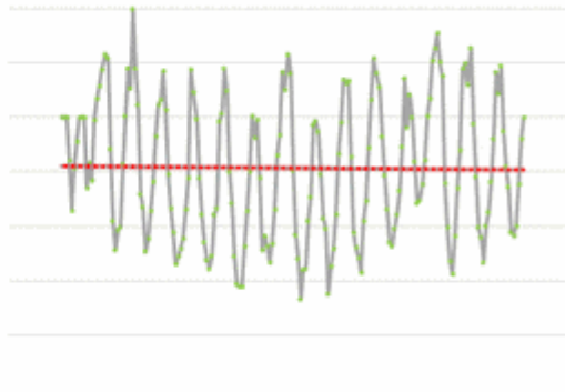
Pegelverlauf Turtle head Nordaustralien
