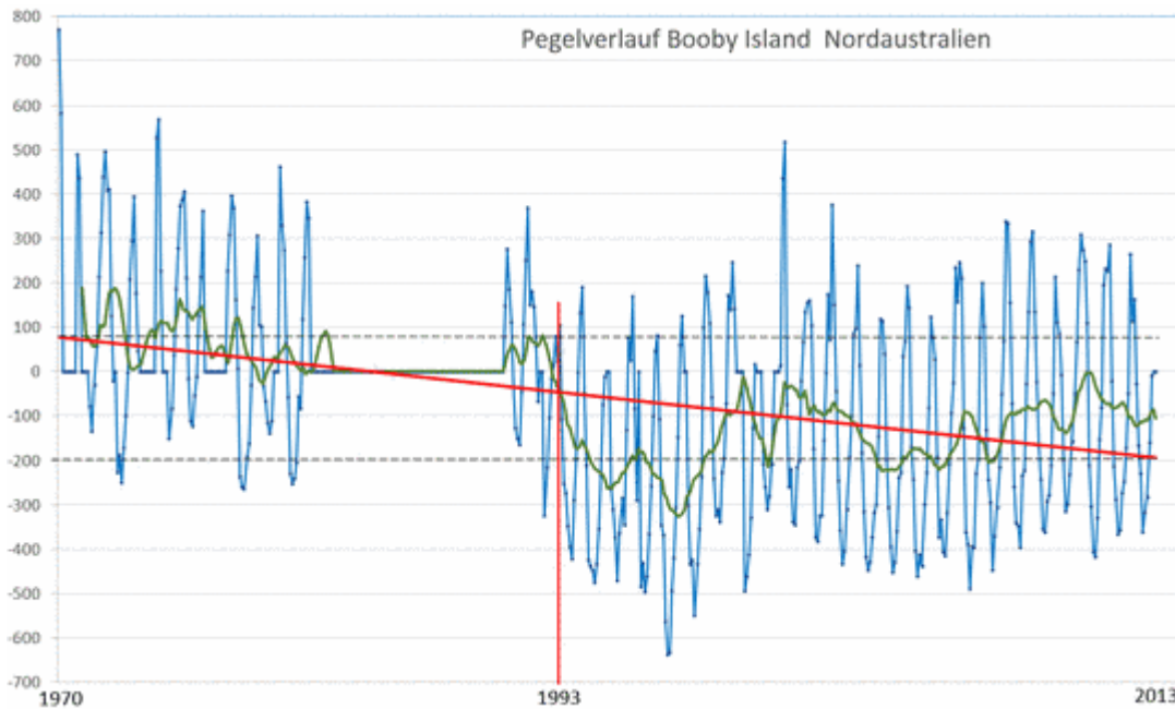
Bild 5, Pegolverlauf von Booby Island mit Regressionsgerade (rot)
