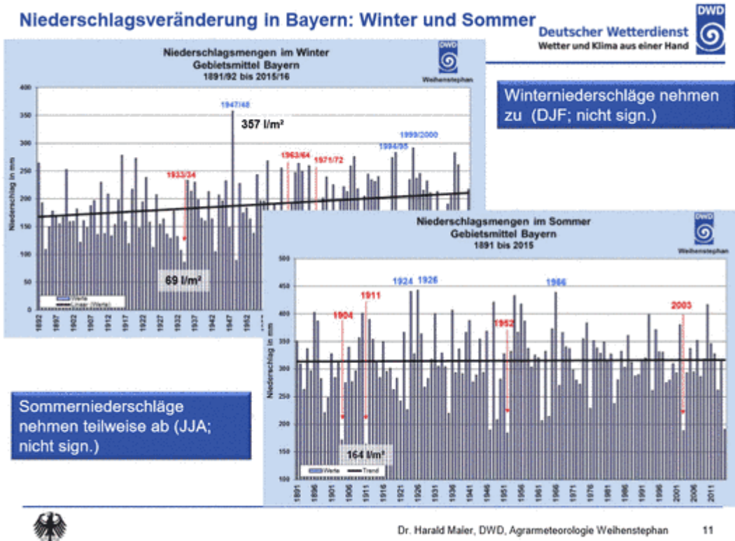
Bild 11 [7] Niederschläge Bayern
