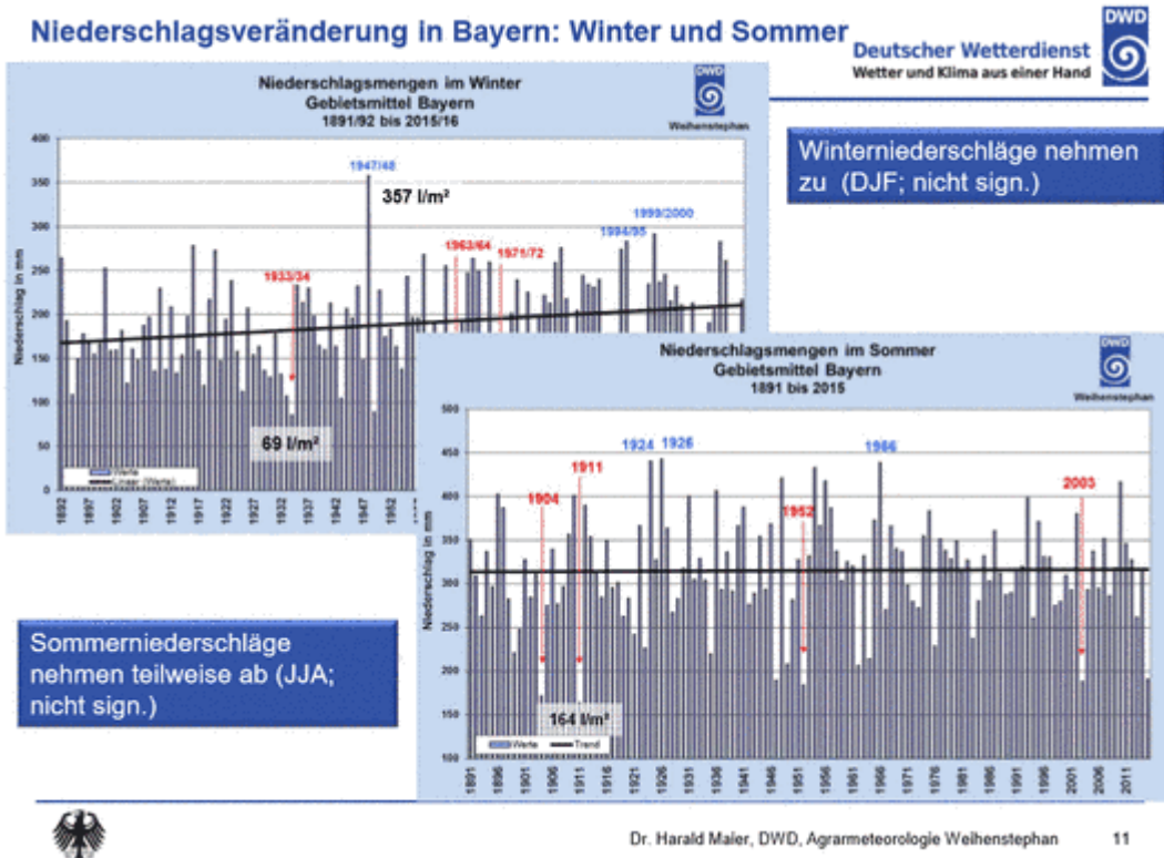
Bild 11 [7] Niederschläge Bayern
