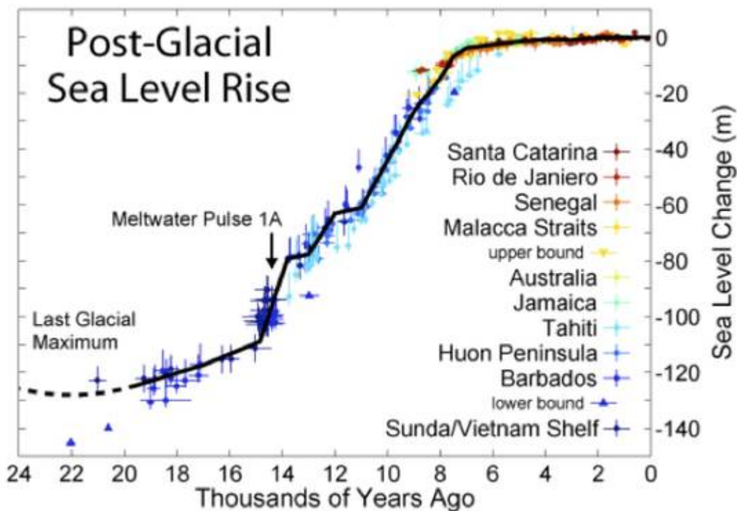
Abbildung 12: Anstieg des globalen Meeresspiegels seit dem Ende der Eiszeit. Deutlich zu erkennen, dass dieser seit ca. 9.000 Jahren nur noch moderat und seit ca. 6000 Jahren sehr moderat ansteigt. (Weitere Details dazu u.a. hier ) Einen wunderbaren Überblick über den gegenwärtigen Stand der Meeresspiegelforschung hatte zuletzt EIKE Autor Kuntz[18] zusammengetragen. Er untersuchte viele Forschungsergebnisse, welche die letzten 10.000 Jahre (Holozän) abdecken
