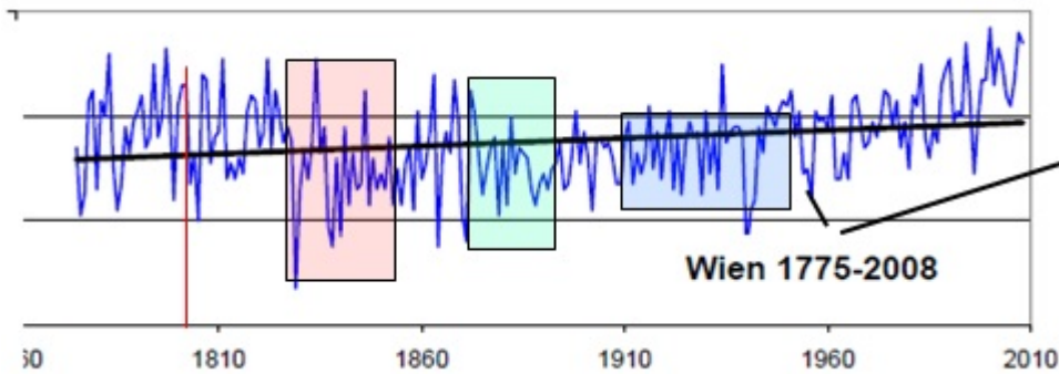
Abb.4: Zu sehen ist der Temperaturverlauf von Wien im Zeitraum von 1775 – 2008, Quelle: Prof. Ewert, EIKE. Die rote Linie gibt den Zeitpunkt des Maximums im Hauptsonnenzyklus an. Bis zu einem Zeitraum von 20 – 30 Jahren nach dem Hauptsonnenzyklus schwanken die Temperaturen am stärksten zwischen warm und kalt (rote Fläche). Bis zu dessen Minimum sind immer noch relativ hohe Temperaturausschläge zu verzeichnen, jedoch auf insgesamt niedrigerem Niveau (grüne Fläche). Unmittelbar vor und nach dessen Minimum ist das Klimasystem sozusagen in seinem eingeschwungenen, kalten Zustand und die Ausschläge sind am geringsten. Vor einem Temperaturanstieg fallen die Temperaturen auf ein relatives Minimum und steigen dann kontinuierlich an (schwarze Linien).
