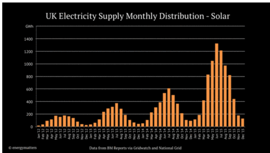
Abbildung 1, Quelle: UK Grid Graphed : Die Verteilung von Solarerzeugung in UK hat sich im Verlauf von 4 Jahren versiebenfacht. Aber 7 mal Tröpfeln im Winter ist immer noch tröpfeln. Die große Menge Energie in diesen teuren Objekten bringt uns gar nichts, wenn wir es am meisten brauchen.
