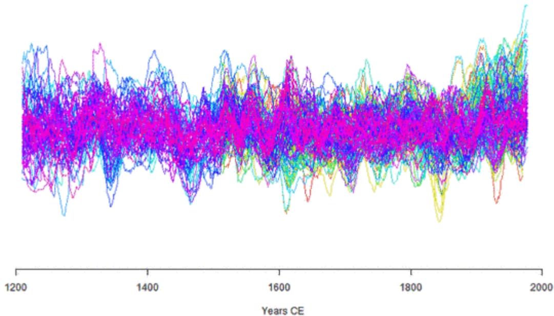
Bild 14.1 Alle Proxys Arctic NAmTR des Projekt PAGES 2k Datensatzes. Quelle: Active viewer for the Pages 2K Proxis
