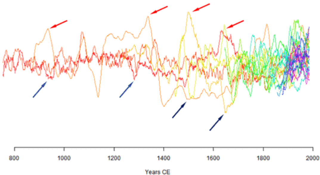
Bild 20 Alle Proxis SAmerica des Projekt PAGES 2k Datensatzes. Quelle: Active viewer for the Pages 2K Proxis
