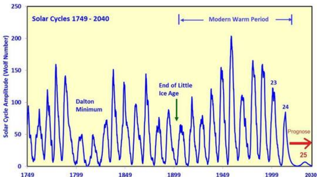
Abb. 9: Verlauf der Sonnenfleckenzahlen seit 1749. Man erkennt die sehr hohe Aktivität in der 2. Hälfte des 20. Jahrhunderts. Der nächste (25.) SCHWABE- Zyklus, der um oder kurz nach 2020 beginnen müsste, könnte extrem schwach ausfallen; diese Prognose ist aber noch sehr unsicher. Quelle der Abb. klimaskeptiker.info vom 25.01.2012, überarbeitet von Stefan Kämpfe
