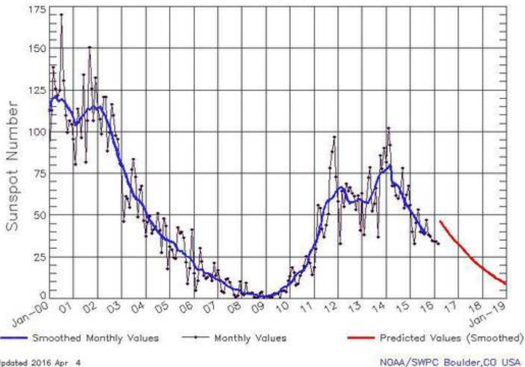
Abb. 7: Monatlicher Verlauf der Anzahl der Sonnenflecken seit Januar 2000 mit Glättung (blau) und Prognose für die nächsten Jahre (rot). Der aktuelle SCHWABE- ZYKLUS Nr. 24 (rechte Bildhälfte) war schon deutlich schwächer als der 23. Zyklus, der sein Maximum kurz nach Beginn des Jahres 2000 hatte. Man erkennt die zu erwartende weiter nachlassende Aktivität (ganz rechts). Datenquelle http://www.swpc.noaa.gov/products/solar-cycle-progression
