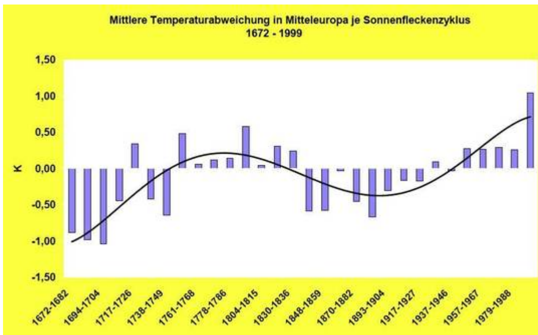
Abb. 1a und 1b: Anomalien der Sonnenfleckenanzahl je SCHWABE- Zyklus (oben) und mittlere Temperaturabweichung in Mitteleuropa je SCHWABE- Zyklus (unten), jeweils mit Polynom- Ausgleichskurven (schwarz). Quelle: H. MALBERG, ehemaliger Direktor des meteorologischen Instituts der FU Berlin. Die Ähnlichkeit beider Verläufe ist unverkennbar; in Phasen mit weniger Sonnenflecken (geringere Aktivität) dominierten negative, in Phasen mit erhöhter Sonnenaktivität hingegen positive Temperaturabweichungen.
