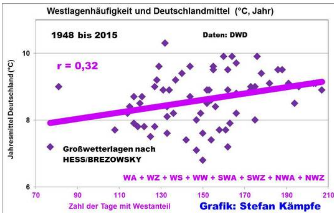
Abb. 5a und 5b: Eine höhere Zonalwindgeschwindigkeit in der mittleren Troposphäre geht mit einer erhöhten Häufigkeit von Großwetterlagen mit Westanteil einher. Mit einem Korrelationskoeffizienten von r=0,59 (Bestimmtheitsmaß knapp 0,35) ist der Zusammenhang signifikant (oben). Mehr Lagen mit Westanteil bedeuten tendenziell höhere Jahresmitteltemperaturen in Deutschland (untere Abb.). Zwar ist der Zusammenhang mit r= 0,32 relativ undeutlich; betrachtet man aber nur den Winter, so ergibt sich im Zeitraum 1948/49 bis 2015/16 ein Korrelationskoeffizient von r=0,72 (Bestimmtheitsmaß knapp 52%), was hoch signifikant ist.
