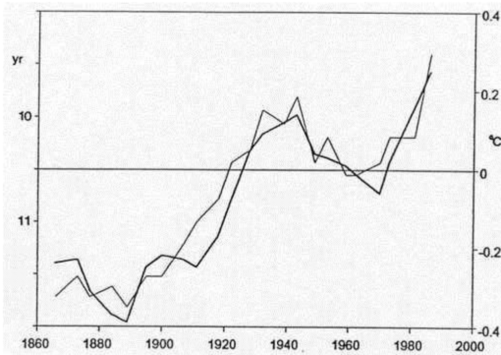
Abb. 2: Enge Korrelation zwischen der an der Erdoberfläche gemessenen Lufttemperatur der nördlichen Hemisphäre (dicke Kurve) und der Intensität der Sonnenflecken-tätigkeit im säkularen Gleissberg- Zyklus (dünne Kurve) nach Friis-Christensen und Lassen. Quelle:
