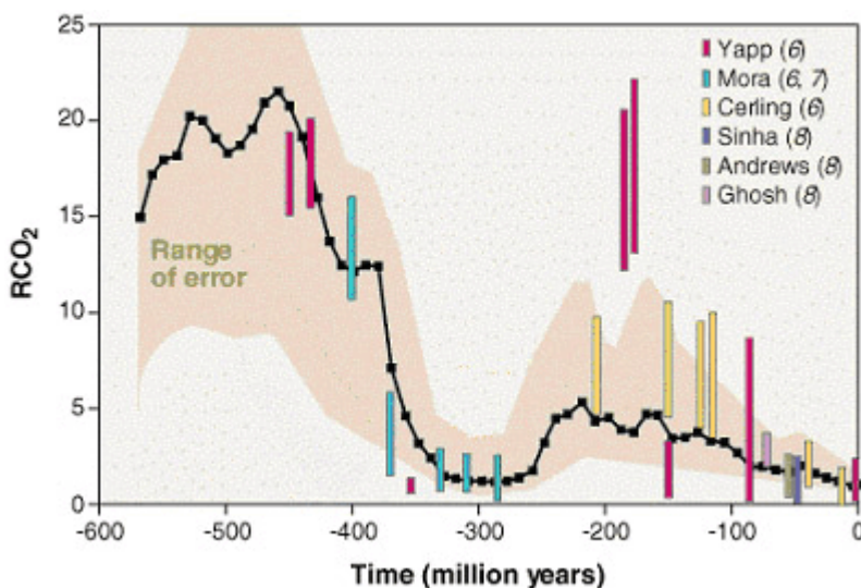
Bild 3. Verlauf des CO 2 -Gehalts im Verlauf der letzten 550 Millionen Jahre im Verhältnis zum vorindustriellen Niveau von rund 300 ppm (RCO 2 = Vielfaches des vorindustriellen Wertes von 300 ppm) (Bild: [CALU])
