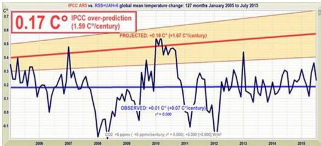
Abbildung 3: Vorhergesagte Temperaturänderung von Januar 2005 bis Juli 2015 mit einer Rate äquivalent zu 1,7 (1,0; 2,3) K pro Jahrhundert (orangefarbener Bereich mit dicker roter Best Estimate-Trendlinie), verglichen mit den beobachteten, nahe Null liegenden Anomalien (dunkelblau) und Trend (hellblau) der realen Welt, gebildet aus dem Mittel der Temperaturanomalien in der unteren Troposphäre nach RSS und UAH.
