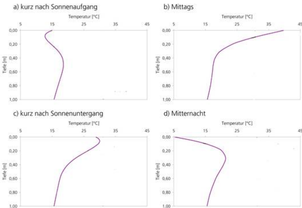
Bild 2. Tagesgang der Temperaturprofile im Boden zwischen Oberfläche und 1 m Tiefe an einem typischen Sommertag [BAYE]
