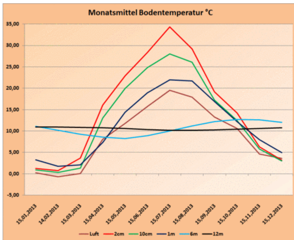
Bild 3. Jahresgang der Temperatur in der Luft sowie im Erdboden im Jahre 2013. Bei 12 m ist faktisch nur noch der Gesamt-Jahreseinfluss zu erkennen (Daten: WIKI und PIK, Grafik: Autor)
