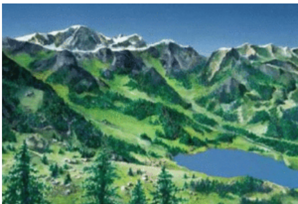
Bild 10: [18] Der Steinlimigletscher (Schweiz) 1993 mit den Ausbreitungslinien von 1856 (obere) und 1913 (untere)
