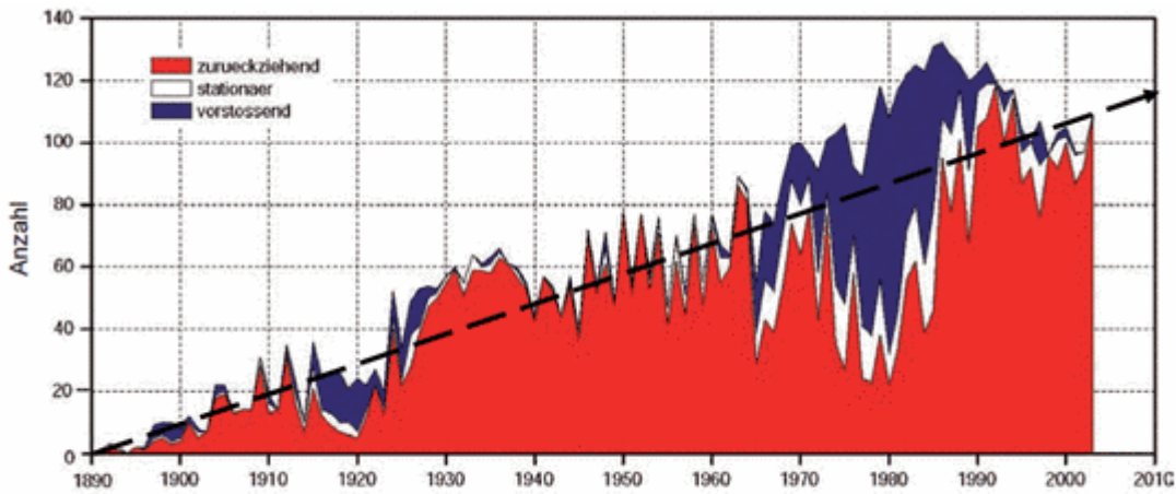
Abb. 6: Längenmessungen an österreichischen Gletschern (Archiv des Österreichischen Alpenvereins)
