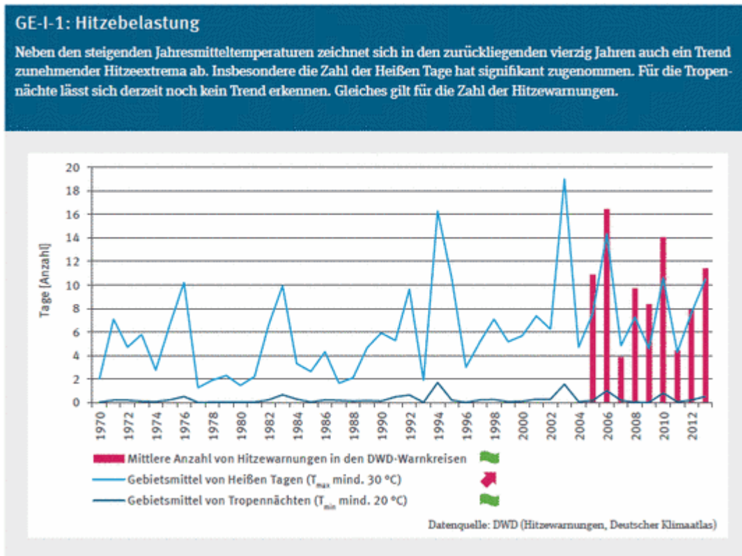
Bild 3: Grafik der Hitzeextreme aus dem Uba-Bericht 2015[3].
