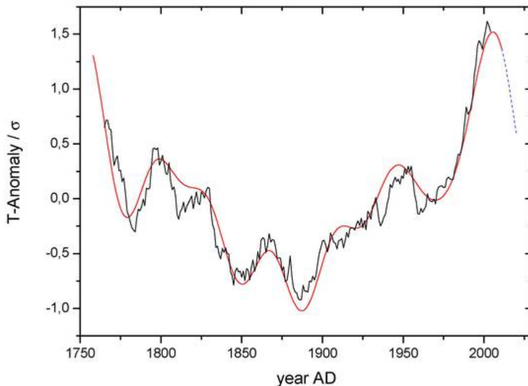
Abb 2 Temperaturverlauf (schwarz; 15 year running mean) von 6 historischen
