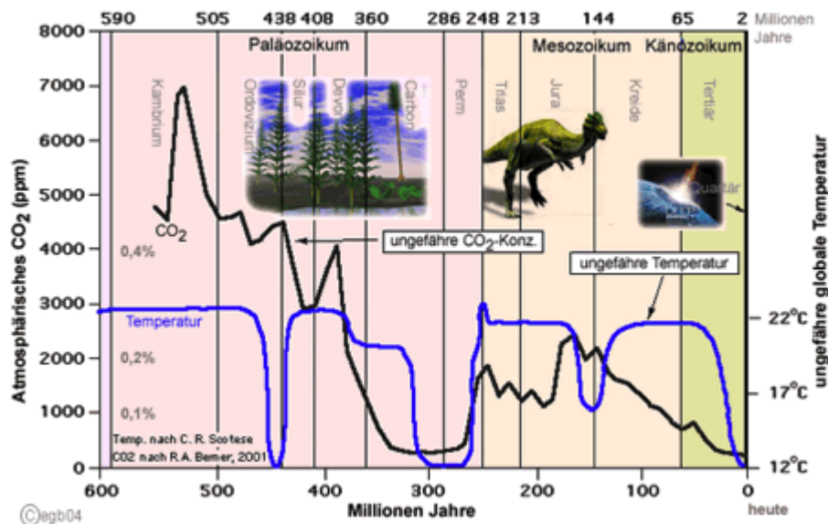
Abb 1 CO 2 und Temperaturverlauf über viele Mio Jahre.
