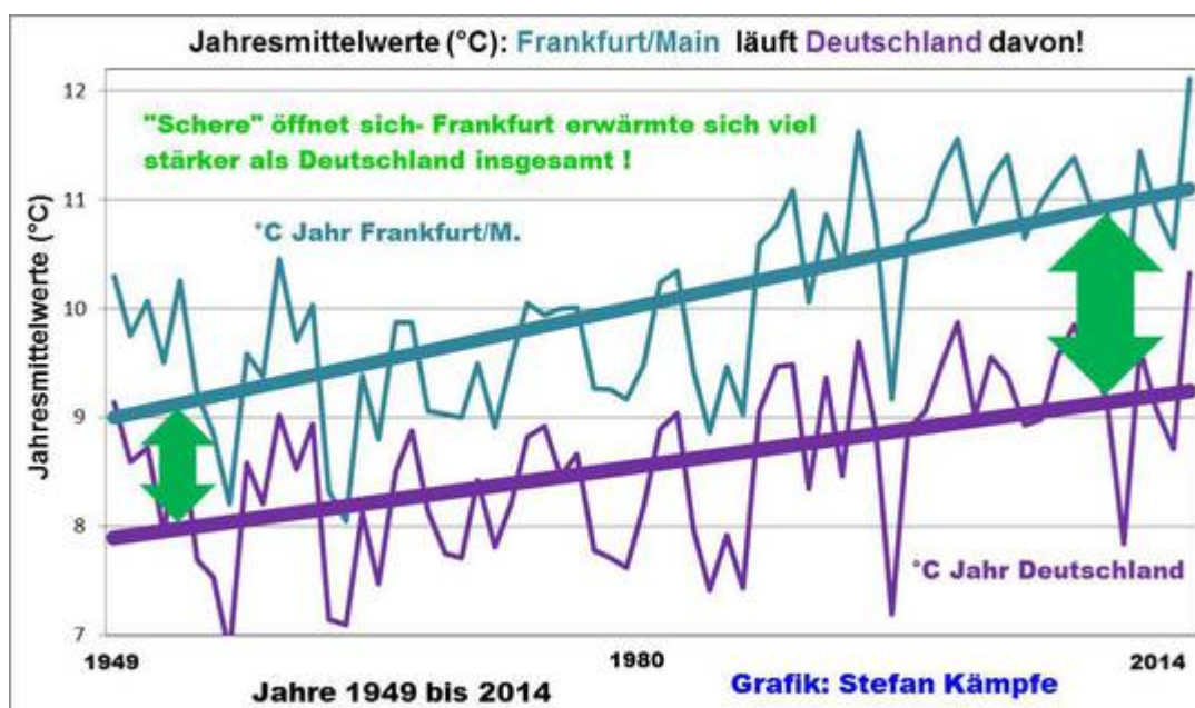
Abb. 8: Die „Schere“ zwischen den linearen Temperaturtrends von FFM (oben) und dem Deutschlandmittel (unten) öffnete sich. Am Anfang der 1949 beginnenden Messreihe war FFM etwa 1,1K wärmer als das Deutschland- Mittel; heuer sind es etwa 1,9K.
