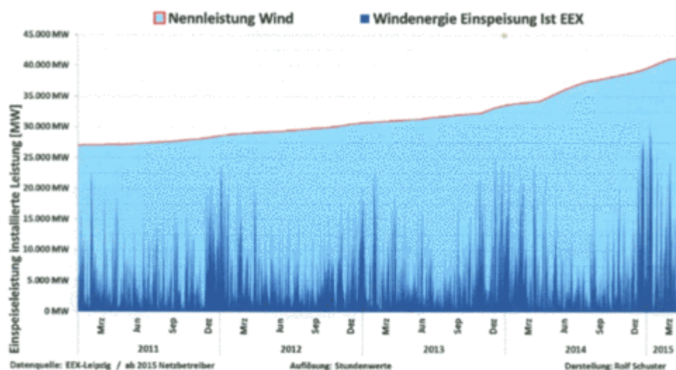
Bild 2: Entwicklung der Windenergie in Deutschland 2011 bis März 2015
