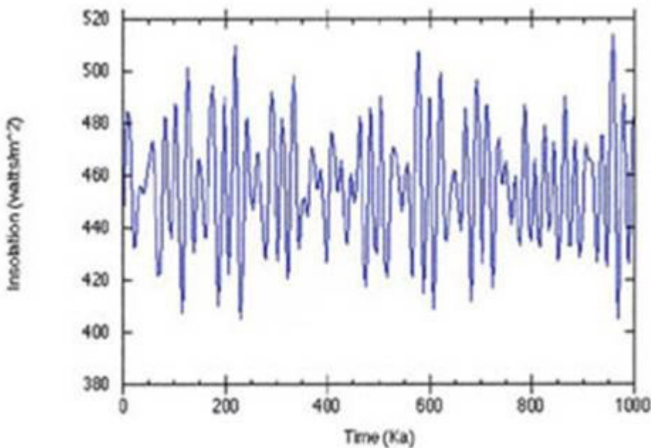
Abbildung 2: Variationen der Einstrahlung (einfallende Solarstrahlung) auf 65^\circ\text{N} .
