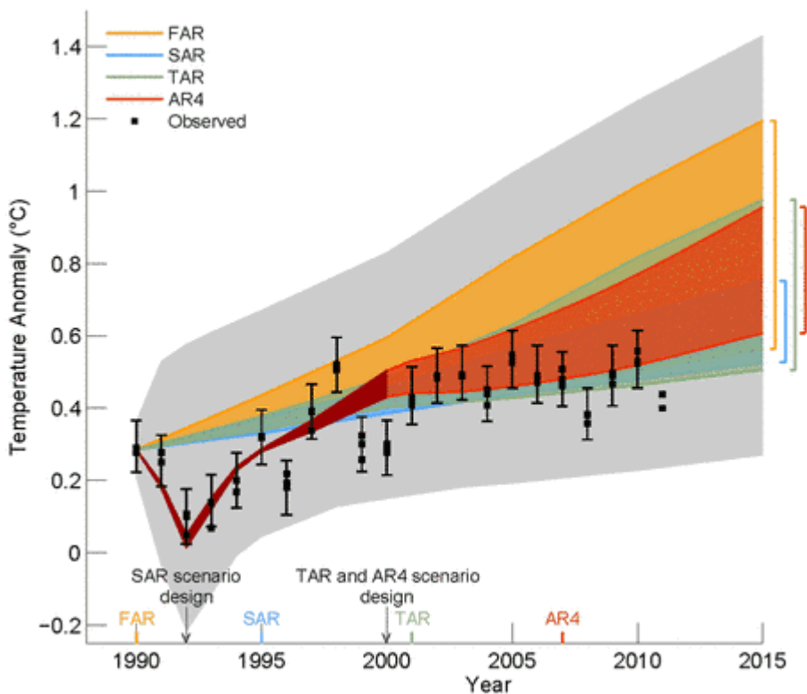
Abb 2: Die derzeit beobachteten Temperaturen (schwarze Punkte) liegen unterhalb der Konfidenzintervalle aller Temperaturprojektionen, die in den ersten 4 IPCC Berichten veröffentlicht wurden (FAR, SAR, TAR AR4). Quelle: 2nd order draft of AR5. The Washington Times, Dec. 18th 2012: Editorial: Chilling Climate-Change News. New leak shows predictions of planetary warming have been overstated.
