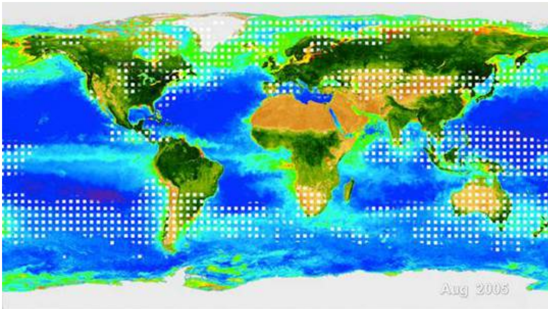
Bild 3 Grün sind die Zonen mit viel Pflanzenwuchs. Im Sommer erreichen die Kohlendioxid-Konzentrationen über Nordamerika, Europa und Asien ein Minimum. Nur wenige weiße Quadrate zeigen dies an.
