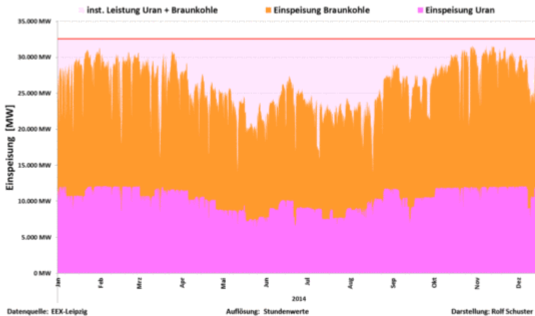
Bild 3: addierte Einspeisung und Nennleistung von Braunkohle und Kernkraftwerken bis zum 16.Dezember
