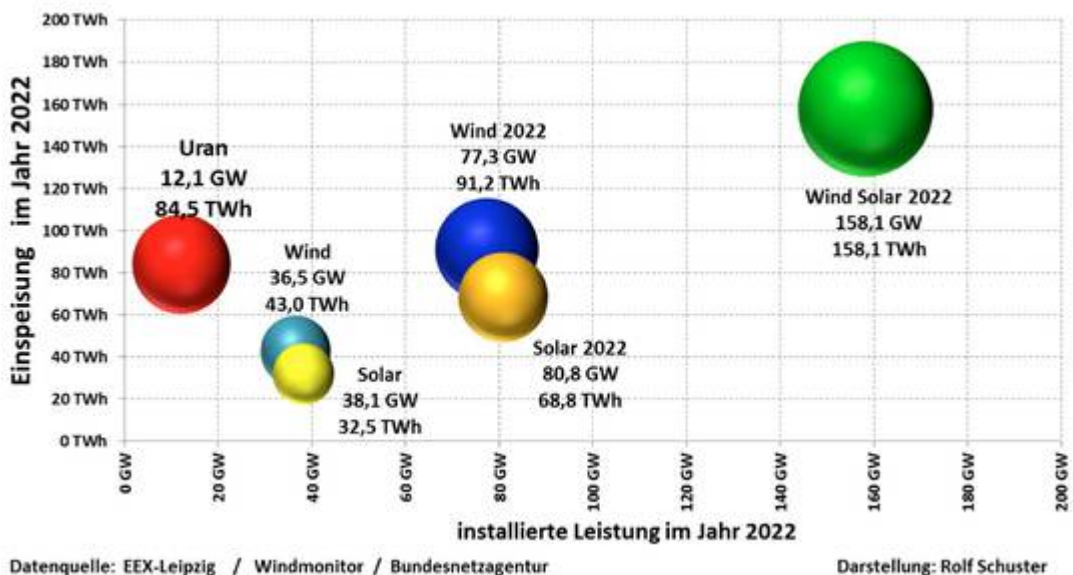
Bild 5: Summe Einspeisung und installierte Leistung im Jahr 2022
