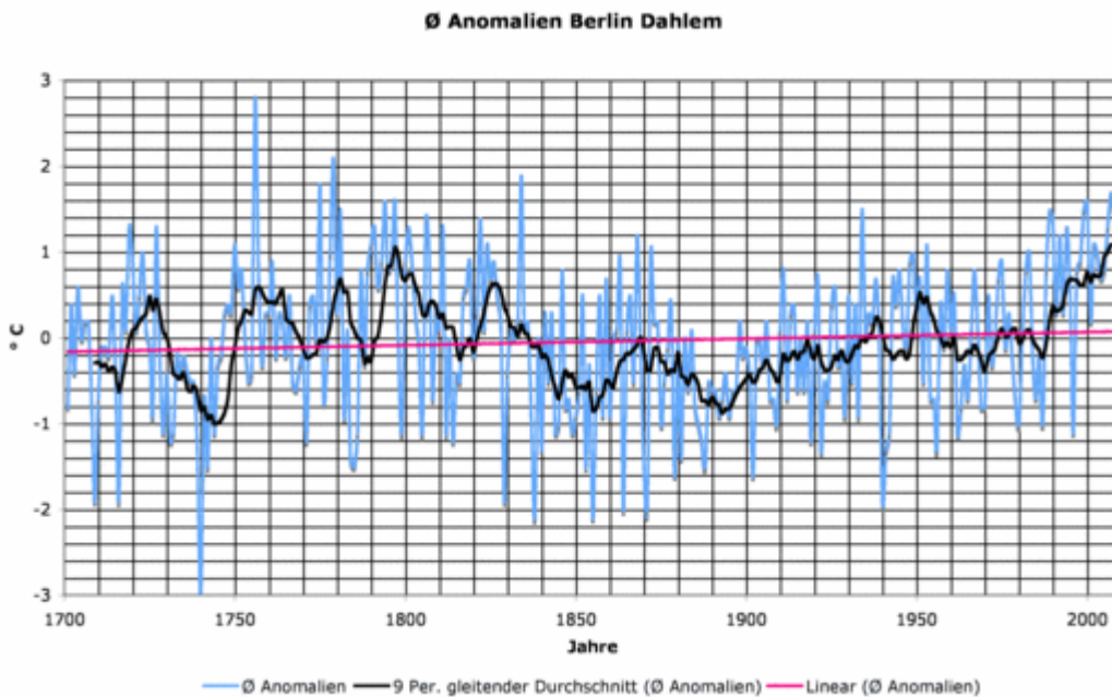
Abb. 1 Temperaturverlauf Berlin & Dahlem 1700 -2008 Quelle: Institut f. Meteorologie FU Berlin; Stand 2009
