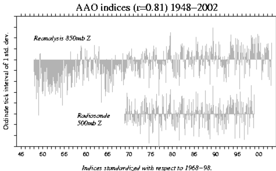
Abb.3 [10] Antarktische Oszillation (AAO)
