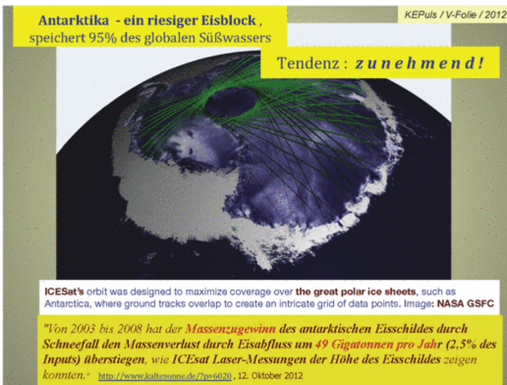
Abb.2 Antarktis-Eiszuwachs [6]
