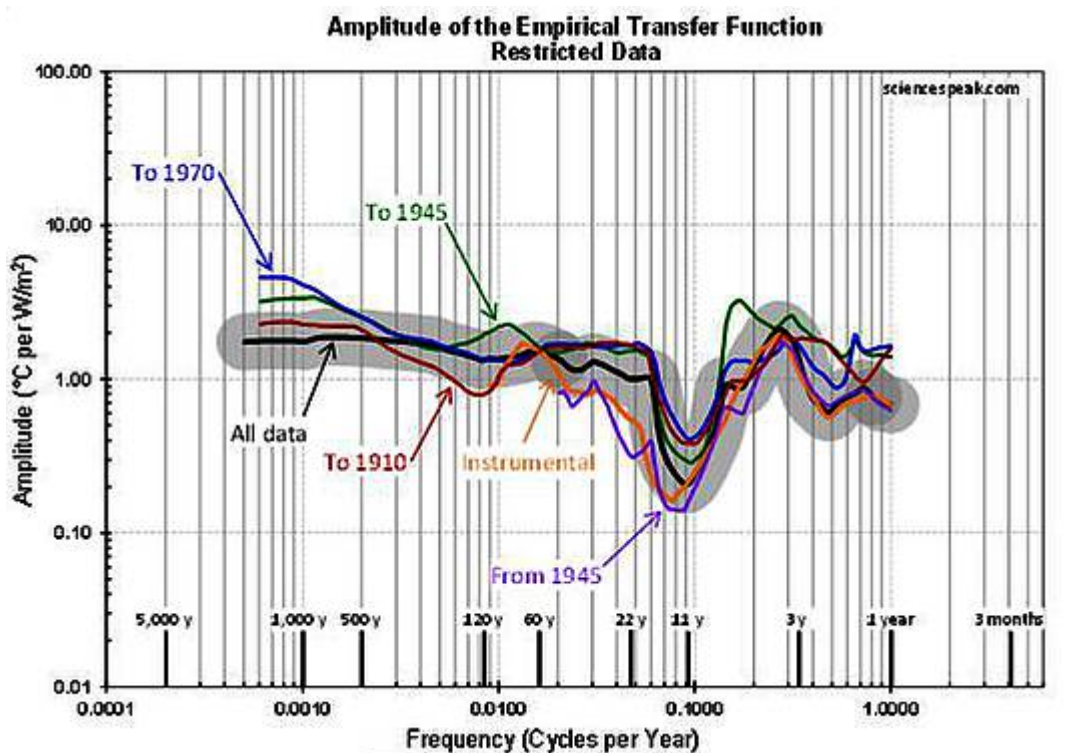
Abbildung 6: Die Amplituden der empirischen Transfer-Funktion, wenn die Daten in der markierten Weise begrenzt werden (das heißt, unter Verwendung einer Sequenz des Datensatzes, der zur Erstellung von Abbildung 5 verwendet wurde). Die schwarze Linie und die graue Zone sind entsprechend Abbildung 5.
