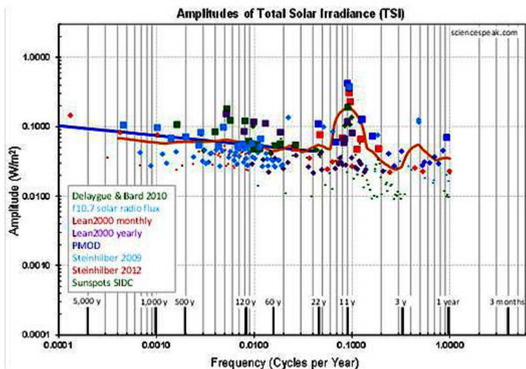
Abbildung 2: Die Amplituden-Spektren der verschiedenen TSI-Datensätze (die Reihe farbiger Punkte) und die geglättete Kurve des Best Fit (orange Linie). Größere Punkte haben mehr Gewicht bei der Glättung. Man beachte die Spitze um
