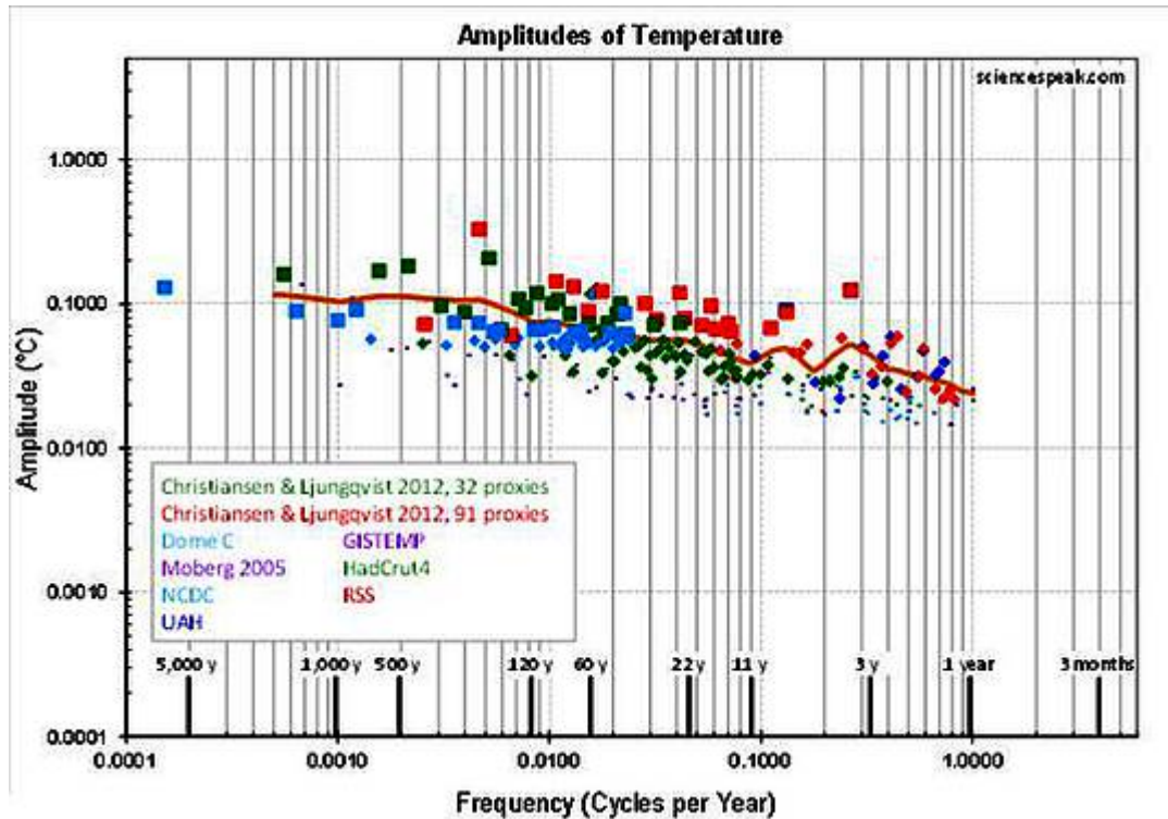
Abbildung 4: Die Amplituden-Spektren der verschiedenen Temperatur-Datensätze (die Reihe farbiger Punkte) und die geglättete Kurve des Best Fit (orange Linie). Größere Punkte haben mehr Gewicht bei der Glättung.
