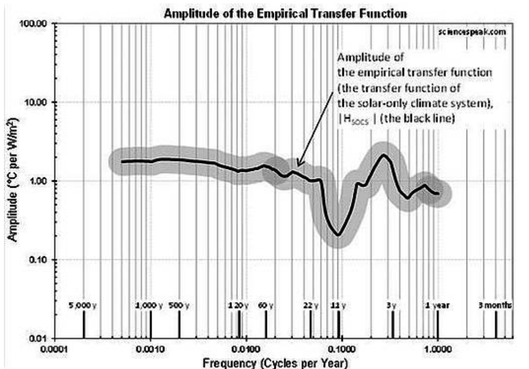
Abbildung 5: Die Amplitude der empirischen Transfer-Funktion. Die graue Zone ist ein graphisches Hilfsmittel, um es einfacher zu machen, Orte auf und zwischen den Graphiken zu beurteilen und zu vergleichen – weil sie genau am gleichen Ort in allen Diagrammen in diesem Projekt liegen.
