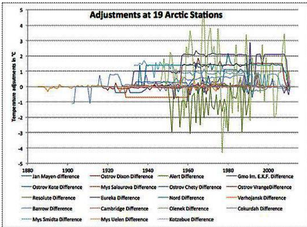
Abbildung 3: Plot aller Anpassungen für alle 19 Stationen
