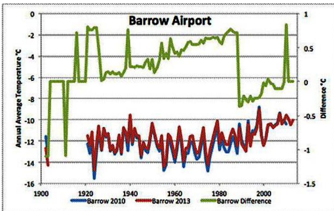
Abbildung 2: Plot der jährlichen Temperatur in Barrow, Alaska,
