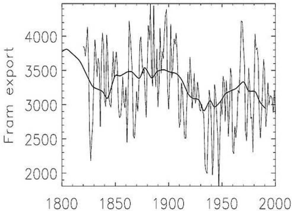
Abbildung 1.7: Variation des Eistransportes durch die Fram-Straße (in Einheiten von \text{km}^3 pro Jahr) und geglätteter Werte der Länge solarer Zyklen (SCL121)(dicke Linie).
