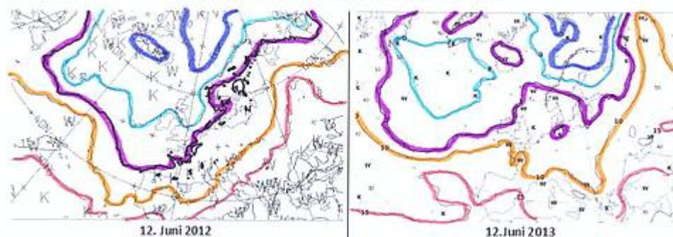
Temperaturverteilung 850 hPa-Niveau 2012 und 2013
