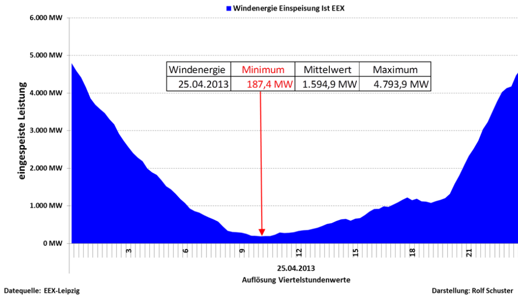
Abbildung 2: Gesamt-Windeinspeisung für den 25.4.13
