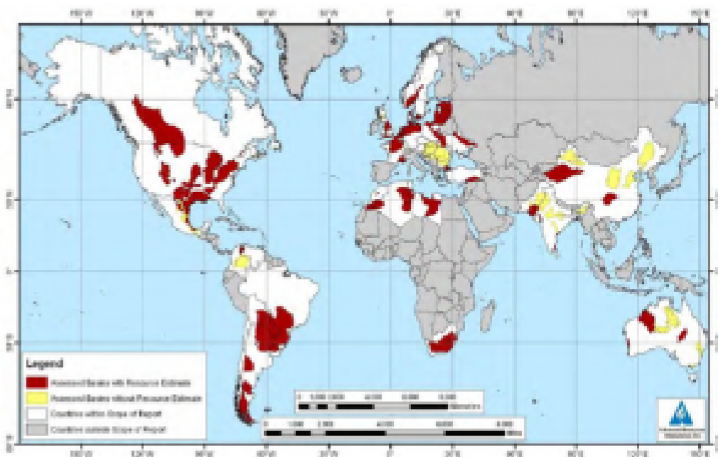
Abbildung 3: Wichtige Schiefer-Lagerstätten der Welt [vii]
