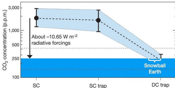
Atmosphärischer CO 2 -Verlauf während der Zeit vor dem Sturtischen Schneeball-Ereignis
