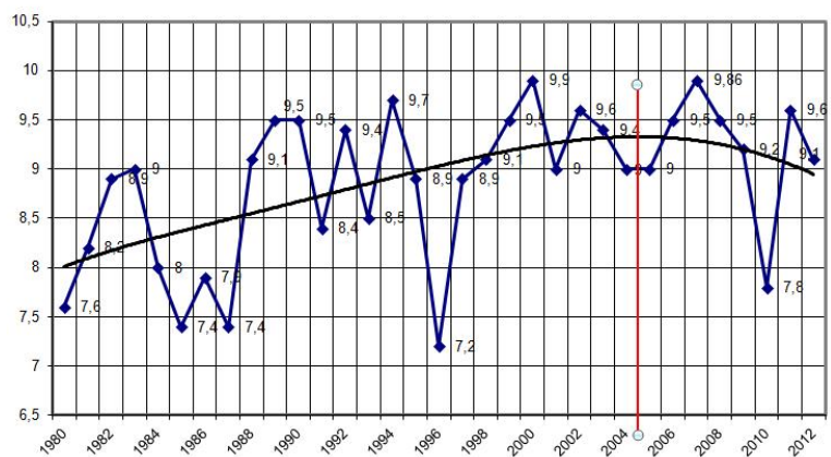
Deutschlandtemperaturen 1980 bis 2012
