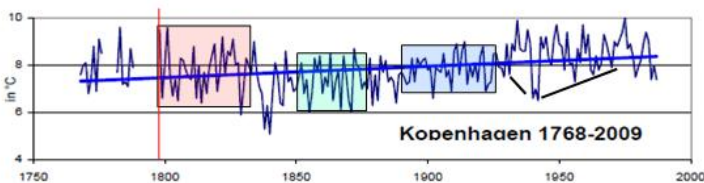
Abbildung 15, Quelle: Prof. Ewert, EIKE, zeigt den Temperaturgang von Kopenhagen im Zeitraum von 1768 – 2009. Die rote Linie gibt den Zeitpunkt des Maximums im Hauptsonnenzyklus an. Bis zu einem Zeitraum von 20 – 30 Jahren nach dem Maximum des Hauptsonnenzyklus schwanken die Temperaturen am stärksten zwischen warm und kalt (rote Fläche). Bis zum Minimum des Hauptsonnenzyklus sind immer noch relativ hohe Temperaturschwankungen zu verzeichnen, jedoch auf insgesamt niedrigerem Niveau (grüne Fläche). Unmittelbar vor und nach dessen Minimum ist das Klimasystem sozusagen in seinem eingeschwungenen, kalten Zustand und die Ausschläge sind am geringsten. Vor einem Temperaturanstieg fallen die Temperaturen auf ein relatives Minimum und steigen dann kontinuierlich an (schwarze Linien).
