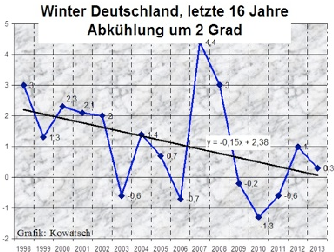
Abbildung 1[1] Winter-Temperaturen 1998-2013 (Dez.-Feb.) in Deutschland
