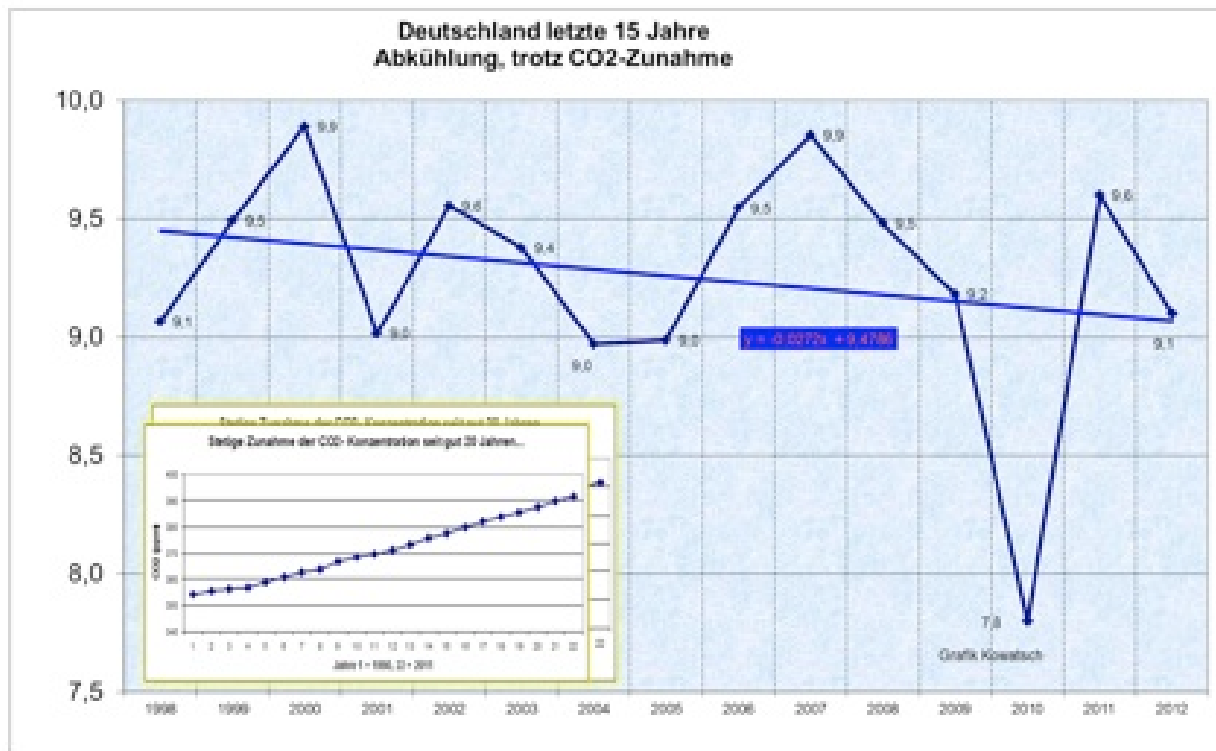
Abbildung 2: Seit 2001 fallen auch die Jahresmittelwerte der Temperaturen in Deutschland deutlich. (Quelle wie Abb. 1)
