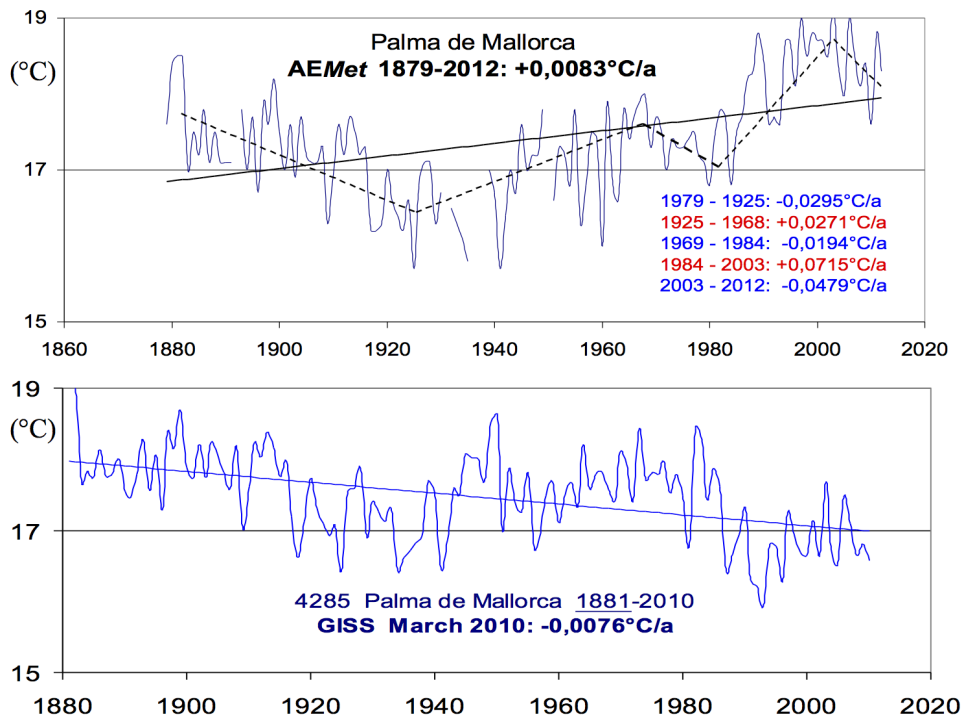
Abb. 2a: Temperaturganglinie Palma de Mallorca, basierend auf den Originaldaten der Station (oben), und den modifizierten NASA-GISS-Daten vom März 2010
