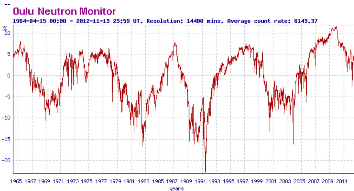
Abbildung 6: Anzahl der Neutronen seit 1964 aus der Oulu-Datenbasis
