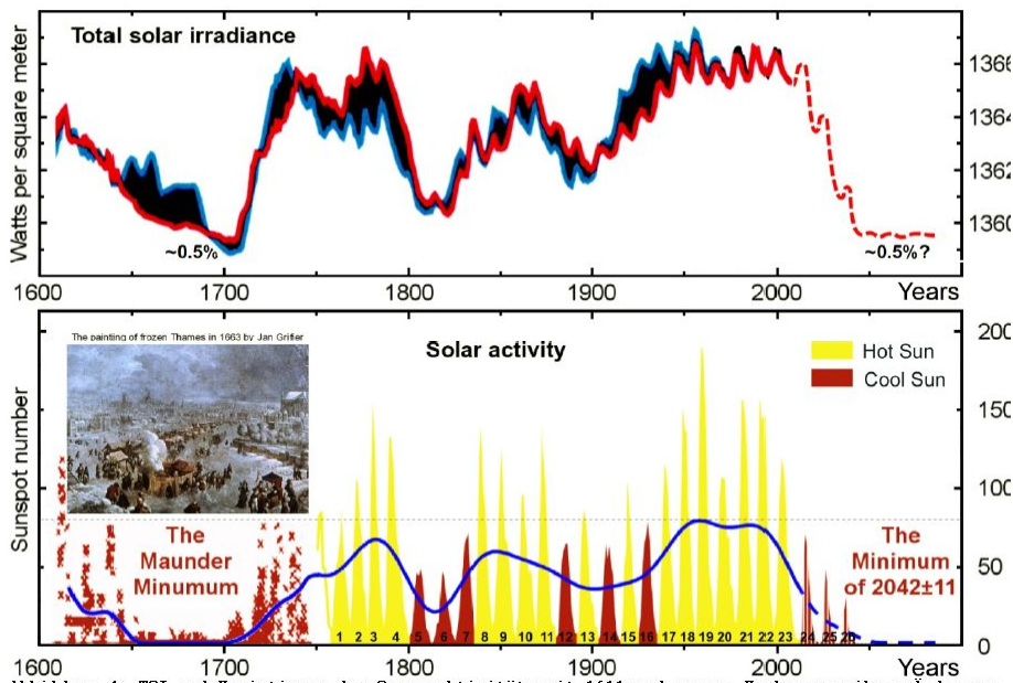
Abbildung 4: TSI und Variationen der Sonnenaktivität seit 1611 und unsere Vorhersage ihrer Änderung (gestrichelte Linien)
