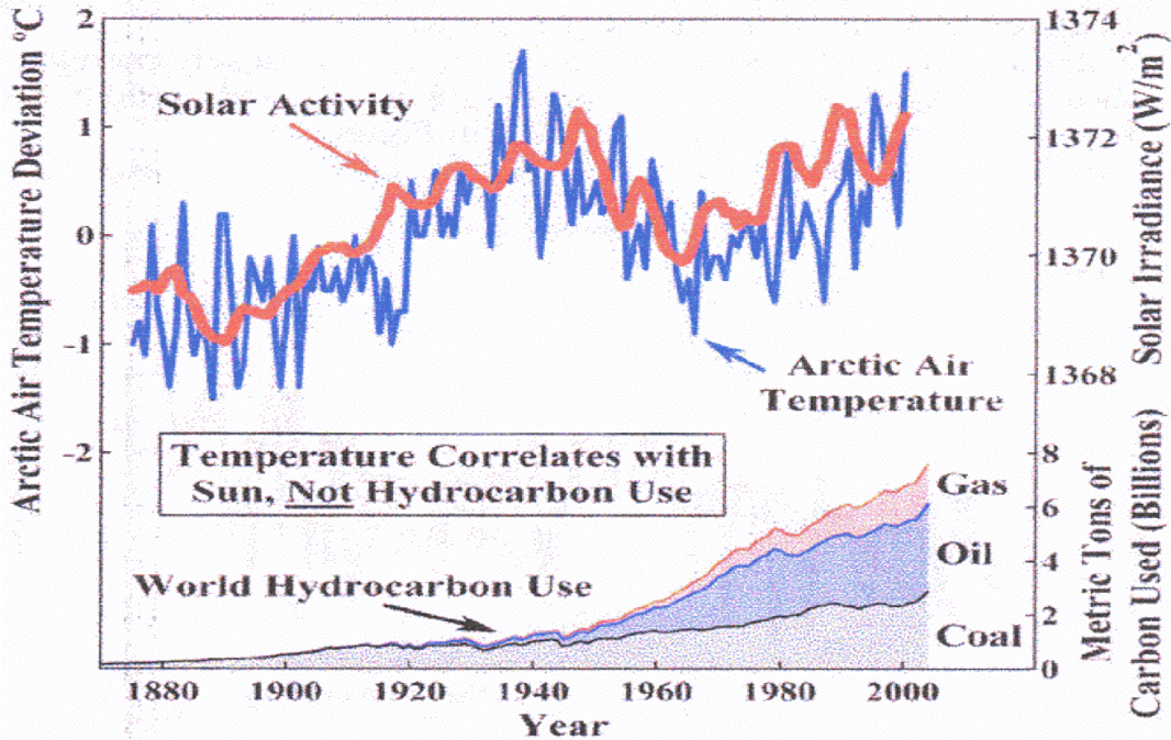
Bild 3: Temperaturentwicklung korreliert mit der Sonnenaktivität, aus [2]
