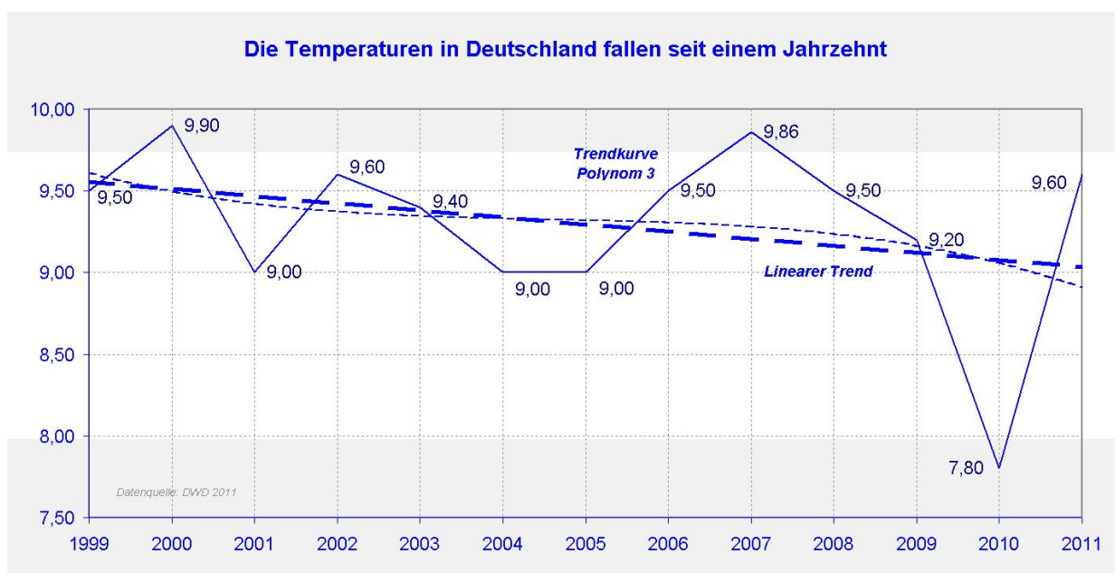
Abbildung 3: Die letzten 13 Jahresmittelwerte in Deutschland seit 1999 waren laut DWD: 9,5 / 9,9 / 9,0/ 9,6/ 9,4 / 9,0 / 9,0/ 9,5 / aufgerundet 9,9/ 9,5/ 9,2/7,8 und 9,6°C. An der blauen Trendkurve sieht man deutlich: Wir haben in Deutschland einen Temperaturrückgang seit über einem Jahrzehnt. Aus diesem Grunde ist auch die Überschrift der neuen DWD-Grafik, siehe Abb1b grob falsch.
