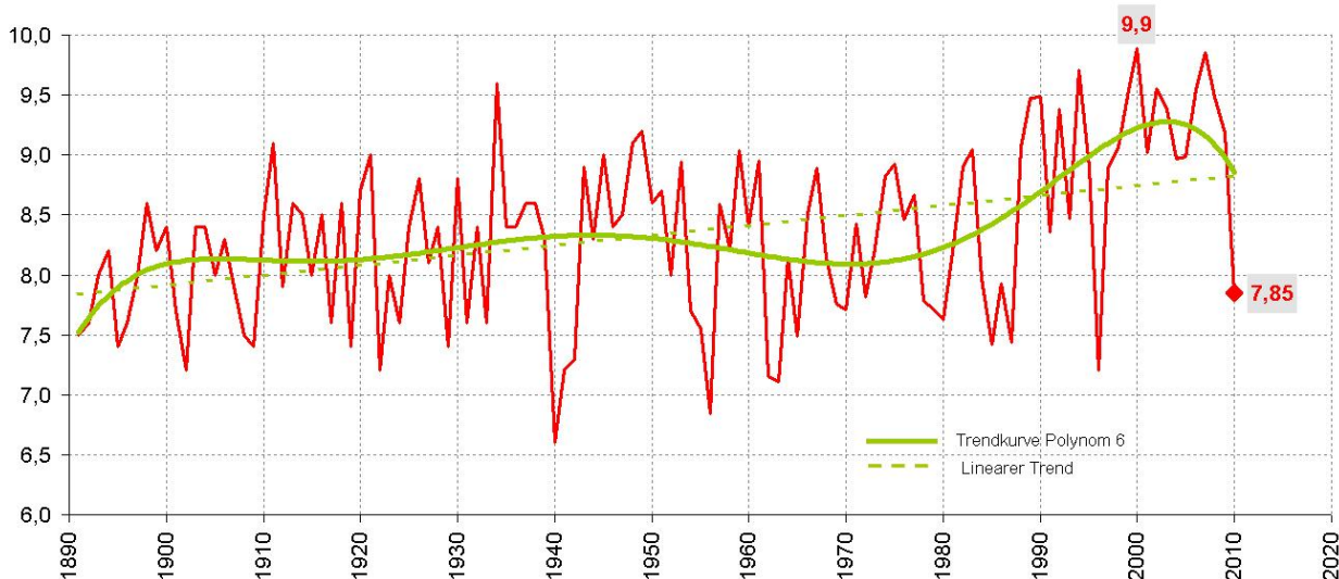
Entwicklung der Deutschlandtemperaturen laut DWD
