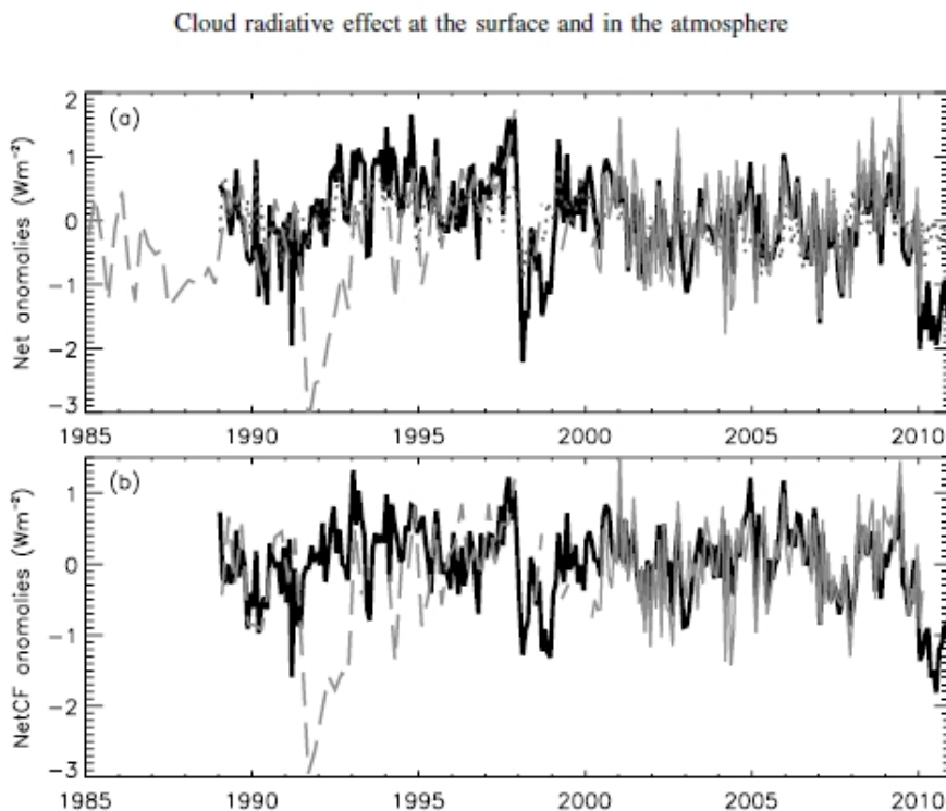
Abbildung 7: Jahreszeitbereinigte monatliche Anomalien (a) der Strahlung und (b) des Strahlungsantriebs der Bewölkung auf fast dem gesamten Globus (60°N bis 60°S) aus der ERA Interim-Analyse, dem ERBS- Übersichtsinstrument und dem CERES-Instrument an Bord von TERRA: ERBS WFOV; CERES Ed2.5Lite; ERA Interim; ERA Interim, clear-sky.
