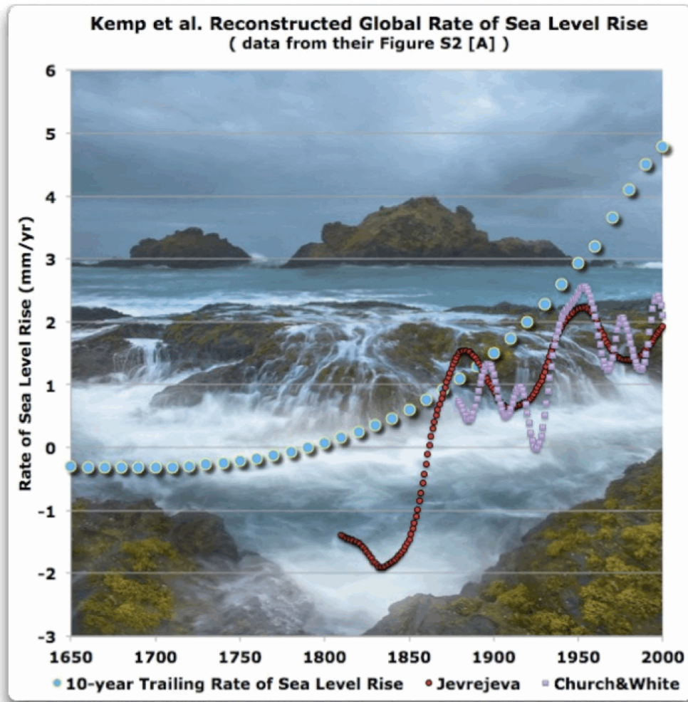
Abb. 3. Die von Kemp 2011 rekonstruierte Rate des globalen Meeresspiegelanstiegs von 1650-2000. Dazu die Beobachtungen von Jevrejeva (rote Kreise) und Church and White (violette Quadrate).
