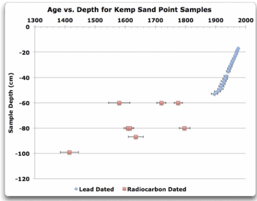
Abb. 5. Alter und Tiefe für die Sand Point Proben im oberen Meter des Bohrkerns. Rote Quadrate zeigen C14 Daten. Horizontale schwarze Balken zeigen die 2-Sigma Ungewissheit (95% Zuverlässigkeits-Intervall).
