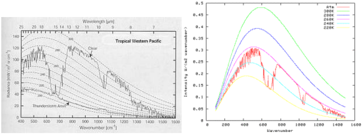
Bild 6: Links das gemessene Emissionsspektrum der Erde (Satellitenspektrum); rechts das mit Hilfe der Strahlungstransportgleichung berechnete Emissionsspektrum
